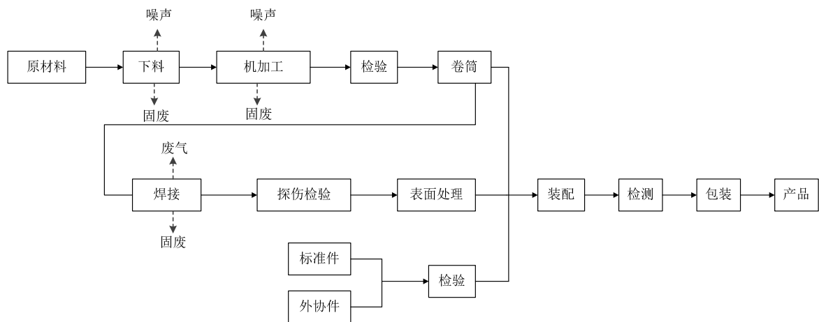
图 2-2 项目工艺流程及产污环节
